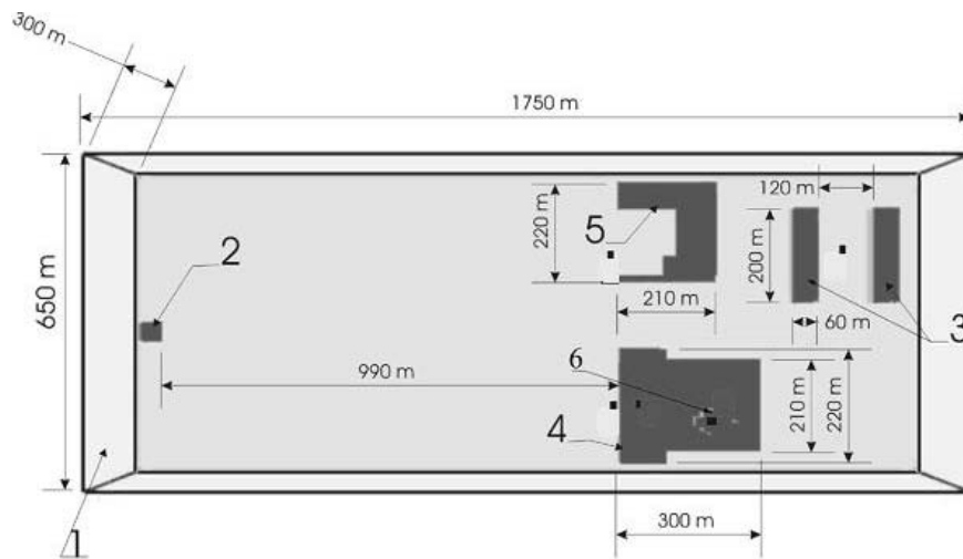
Slika 2. Geometrijska oblika modela (Petelin in Vidmar, 2006).
